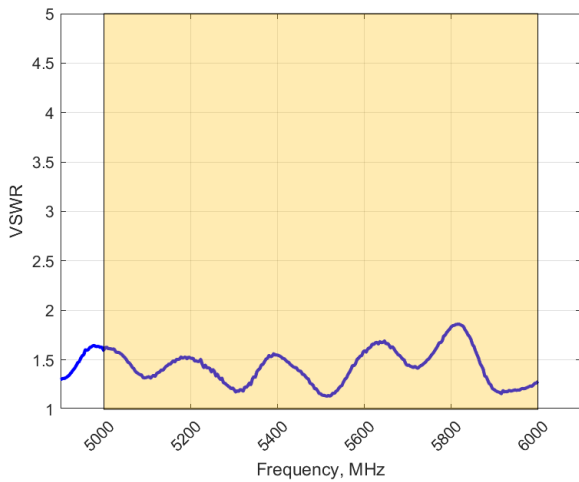
VSWR 5000-6000 MHz
