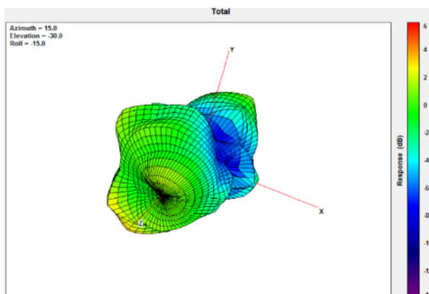
2690MHz
