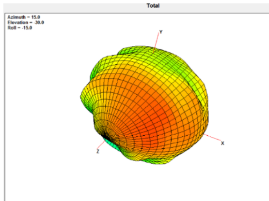
704MHz
