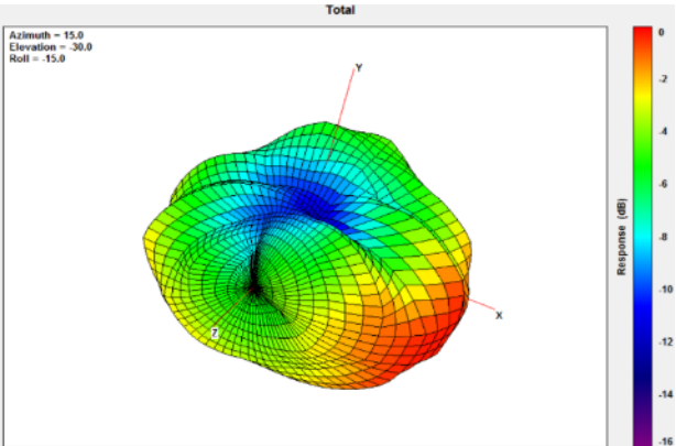
704MHz
