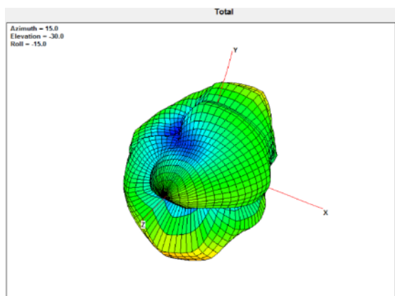
1710MHz
