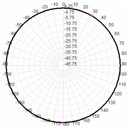
915.0MHz Total(H)
