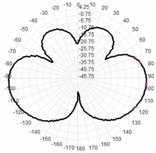
915.0MHz Total(E2)
