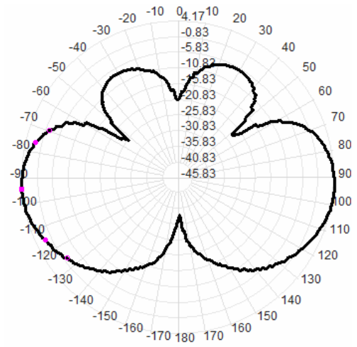
902.0MHz Total(E2)
