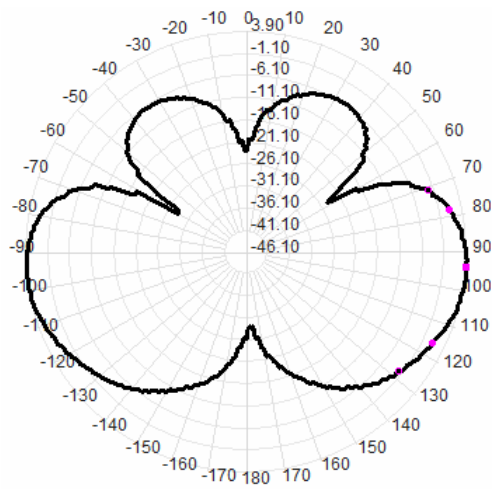
928.0MHz Total(E2)
