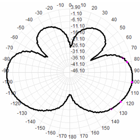
928.0MHz Total(E1)
