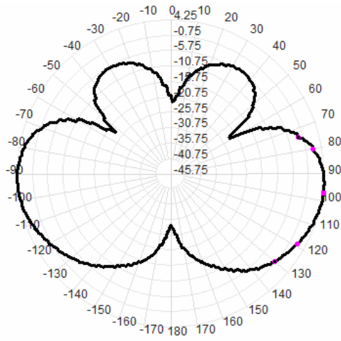
915.0MHz Total(E1)
