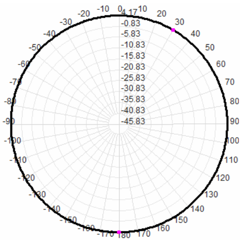
902.0MHz Total(H)
