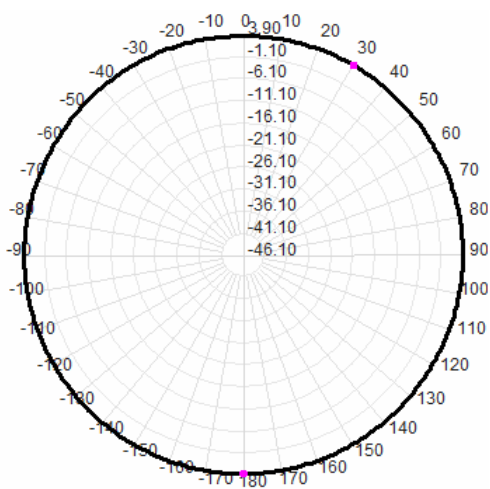
928.0MHz Total(H)
