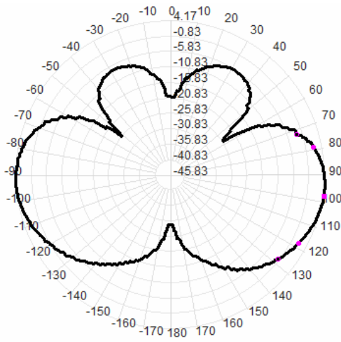
902.0MHz Total(E1)
