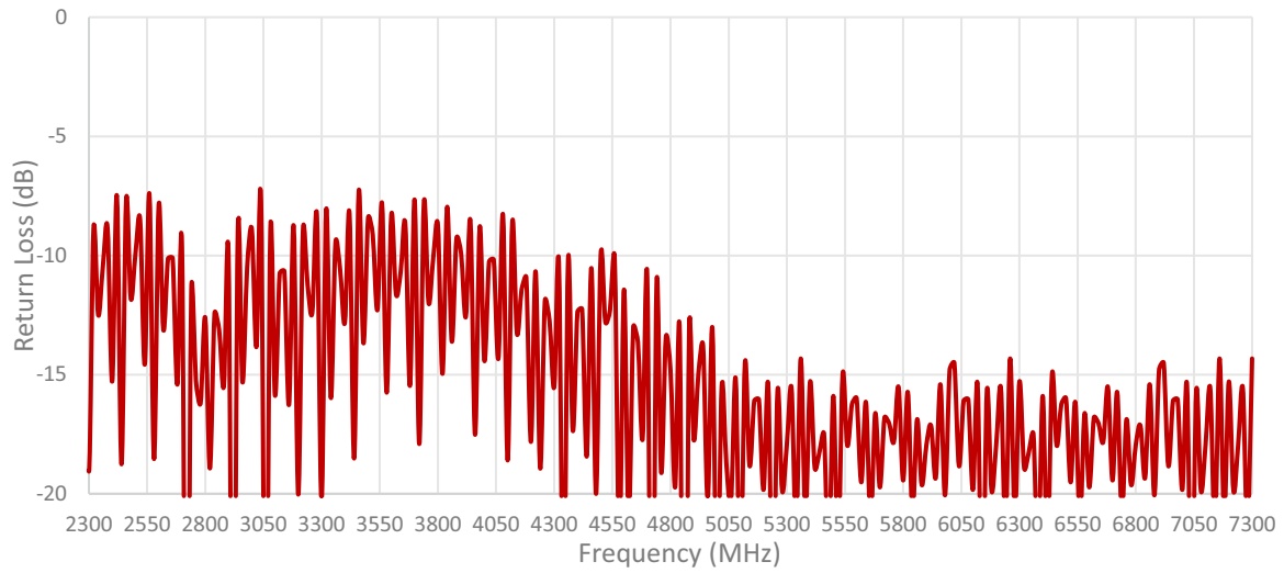
Cable 3: WIFI-6-6E
